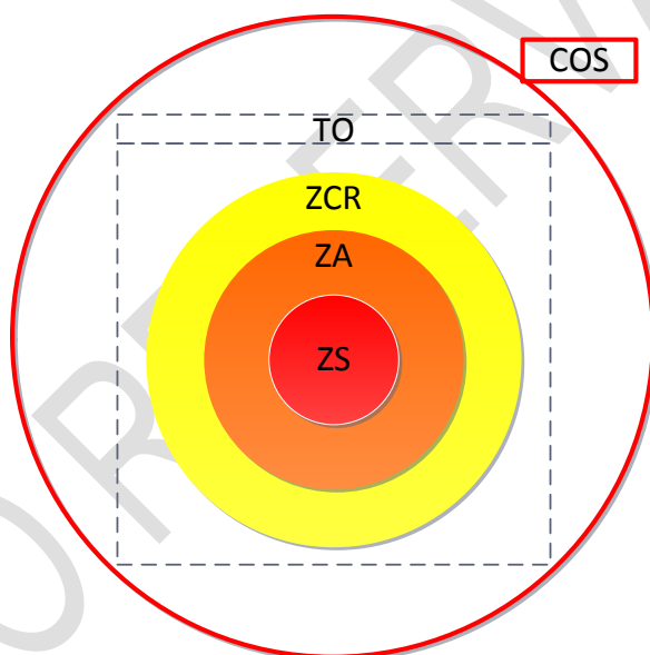
Figura 5 – Diagrama das Zonas de Intervenção
