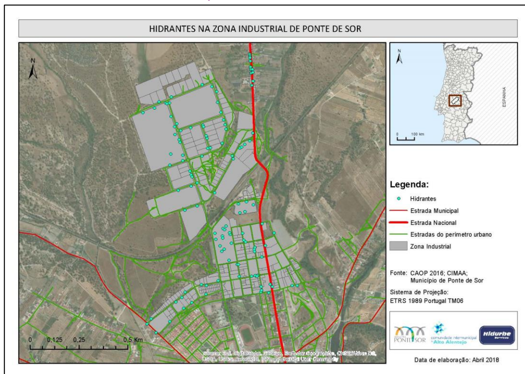
Mapa 3 – Rede de Hidrantes
