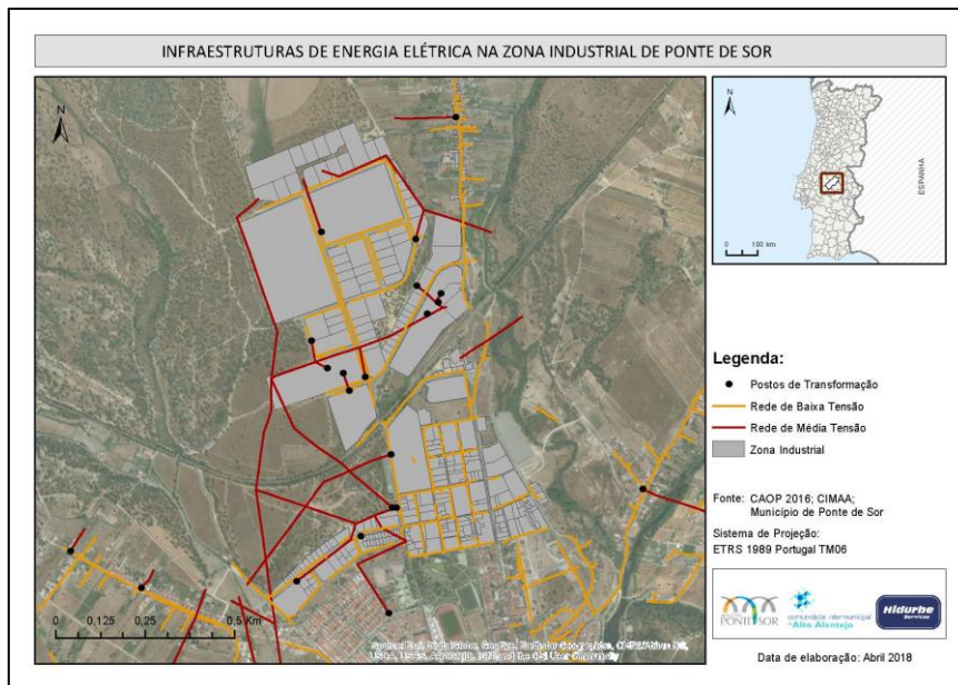
Mapa 4 – Rede de energia elétrica
